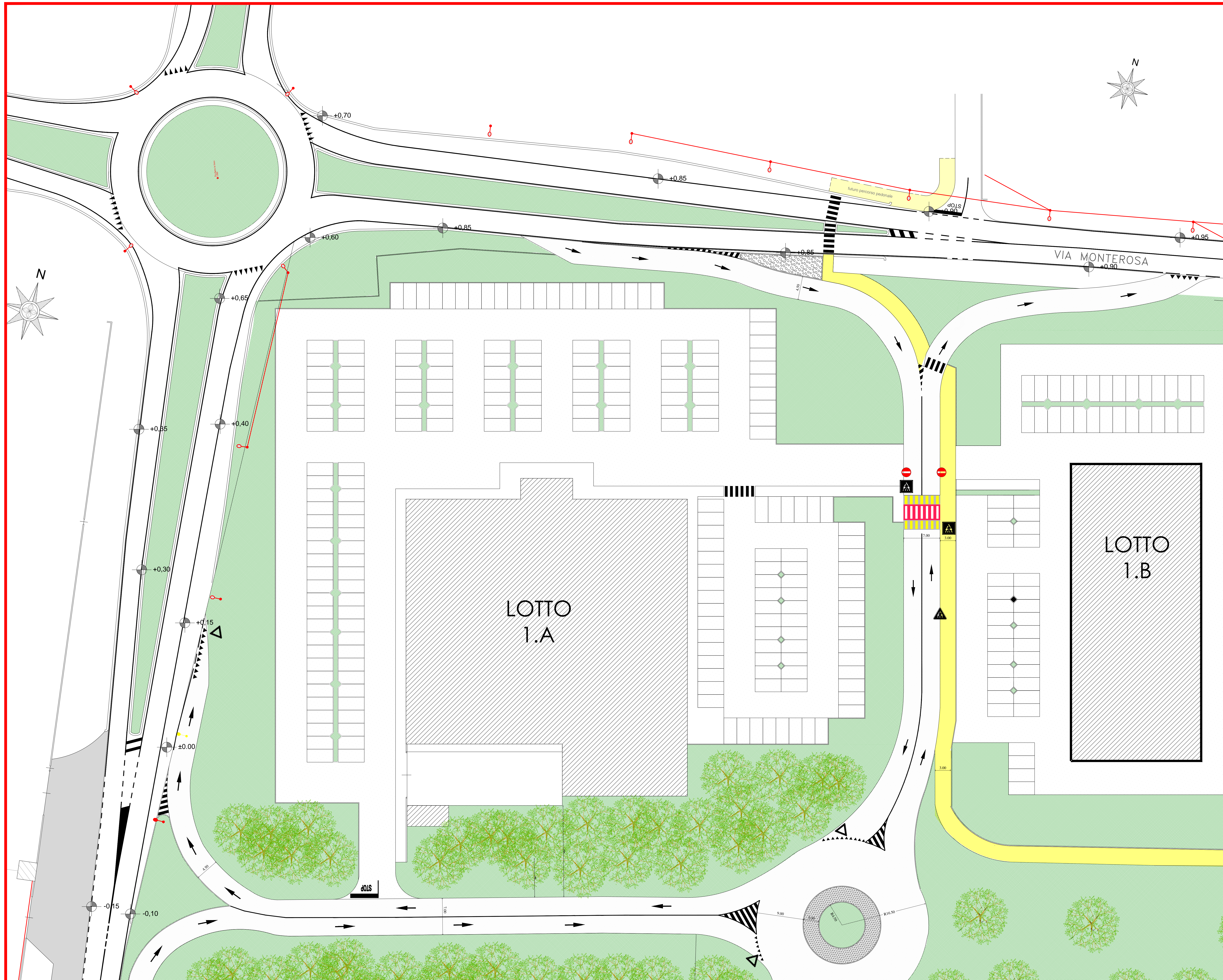
PLANIMETRIA GENERALE DI PROGETTO - SEGNALETICA STRADALE - INQUADRAMENTO 1 - SCALA 1:250
